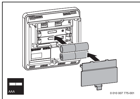
Bild 4 Batterien einsetzen
