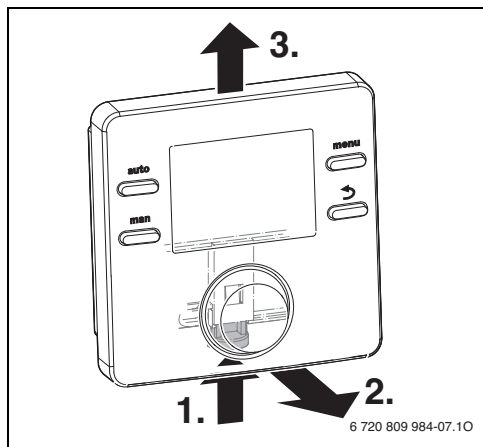
Bild 3 Bedieneinheit abnehmen
