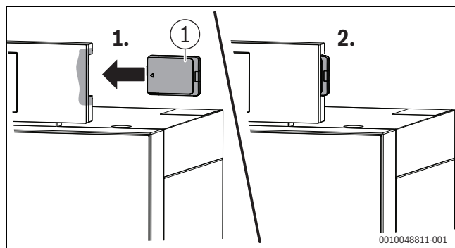
Bild 4 Kommunikationsmodul montieren
