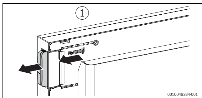
Bild 5 Kommunikationsmodul demontieren
